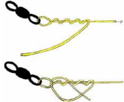
Perukesilmukka-solmu
